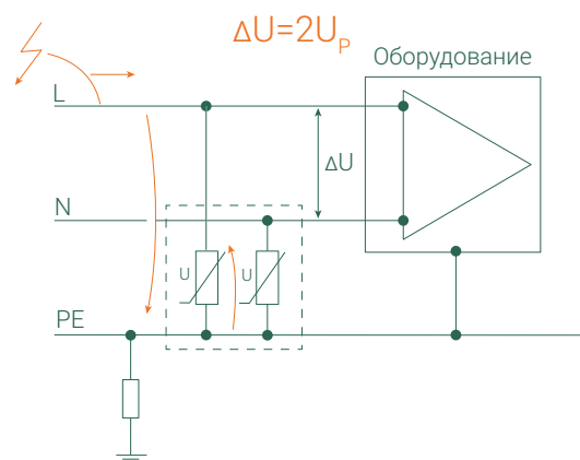
3. Помехи «провод-провод» (противофазные) Схема подключения УЗИП: «2+0»
