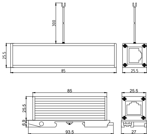
Габаритные размеры
