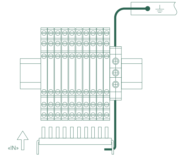
Рис. 30. Заземление группы УЗИП с помощью медного шинпровода
