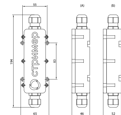
Габаритные размеры
