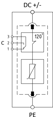
Принципиальная схема
