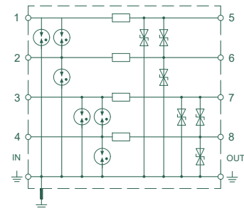
Защита четырех проводников
