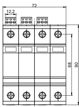
Габаритные размеры
