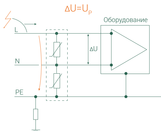
1. Помехи «провод-провод» (противофазные) Схема подключения УЗИП: «1+1»
