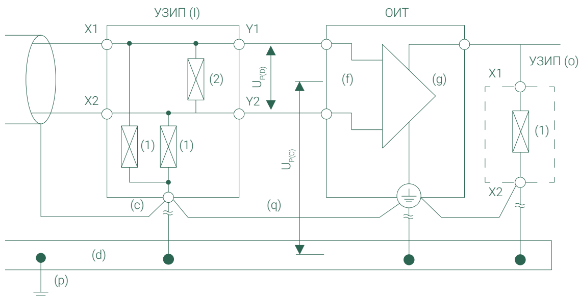
Рис. 24. – Пример защиты ОИТ со стороны питания (g) и передачи данных (f) (I) – информационный УЗИП, (O) – силовое УЗИП, (1) и (2) – компоненты УЗИП для защиты от синфазных и дифференциальных помех соответственно, X1, X2 – выходы УЗИП со стороны источника помех, Y1, Y2 – выходы УЗИП с защищенной стороны, U_{P(C)} – уровень ограничения синфазной помехи, U_{P(D)} – уровень ограничения дифференциальной помехи, (c) – точка подключения УЗИП к заземлению, (d) – шина уравнивания потенциалов, (f) – порт данных ОИТ, (g) – порт питания ОИТ, (h) – информационная линия, (p) – проводник заземления, (q) – соединительный проводник
