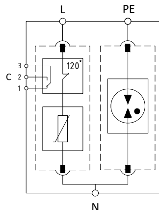
Принципиальная схема
