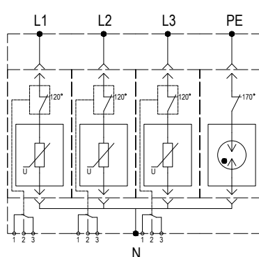
Принципиальная схема
