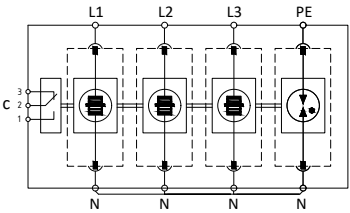
Принципиальная схема
