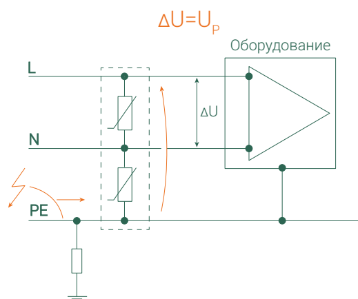
2. Помехи «провод-земля» (синфазные) Схема подключения УЗИП: «1+1»
