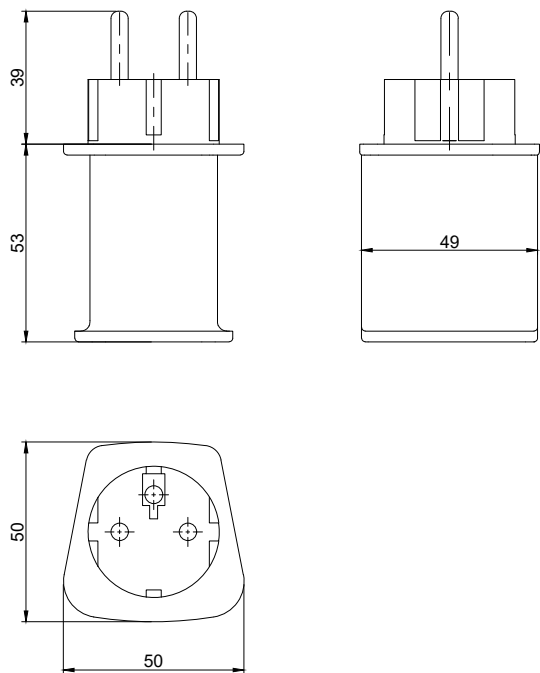
Габаритные размеры
