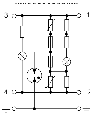
Принципиальная схема
