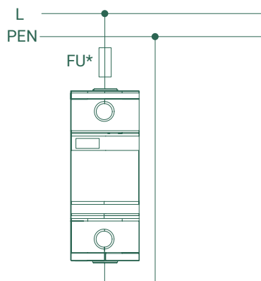
схема подключения «1+0»
