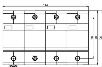
Габаритные размеры
