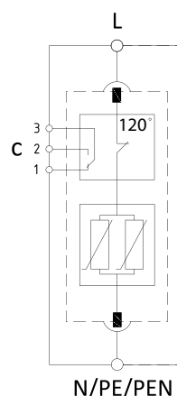
Принципиальная схема
