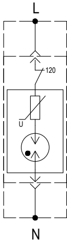
Принципиальная схема
