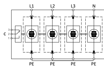
Принципиальная схема
