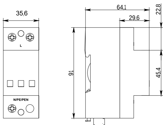
Габаритные размеры
