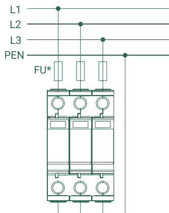
схема подключения «3+0»
