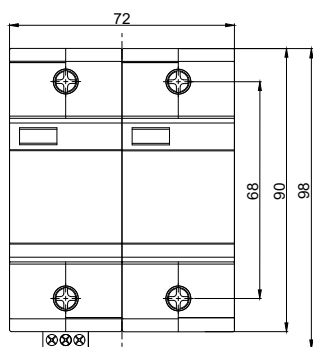
Габаритные размеры
