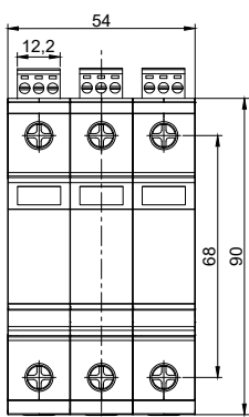
Габаритные размеры
