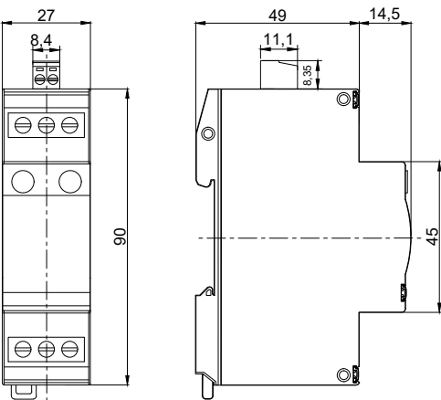
Габаритные размеры
