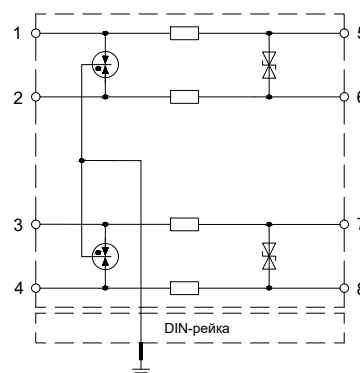
Принципиальная схема
