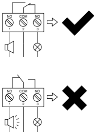
Схема подключения ДС
