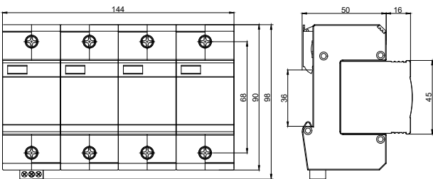
Габаритные размеры
