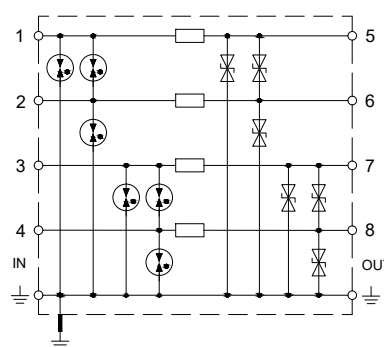
Принципиальная схема
