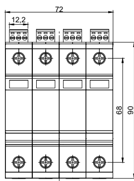
Габаритные размеры
