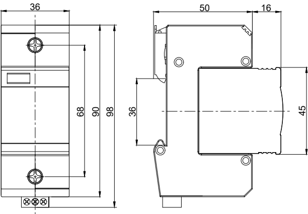
Габаритные размеры
