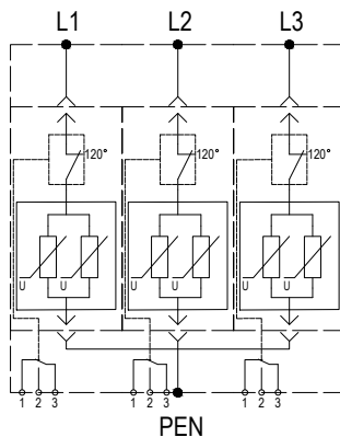
Принципиальная схема
