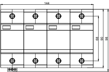
Габаритные размеры
