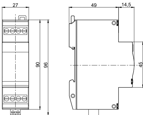
Габаритные размеры
