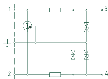
Защита двух проводников
