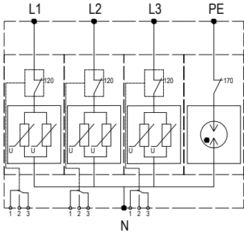
Принципиальная схема
