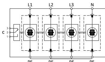
Принципиальная схема
