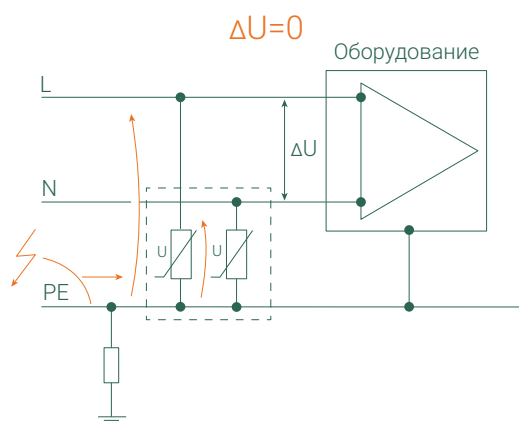
4. Помехи «провод-земля» (синфазные) Схема подключения УЗИП: «2+0»
