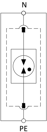
Принципиальная схема
