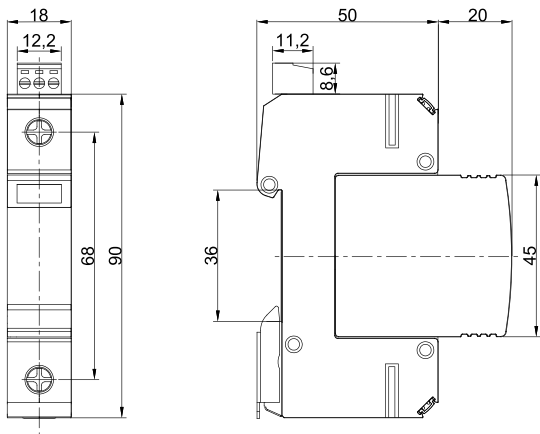
Габаритные размеры
