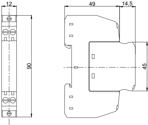
Габаритные размеры
