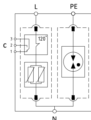
Принципиальная схема
