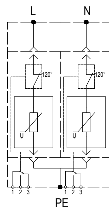
Принципиальная схема
